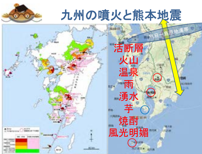
図 12 九州の噴火と熊本地震
