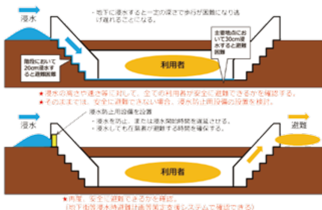
図4-2 安全な避難の確認のイメージ
