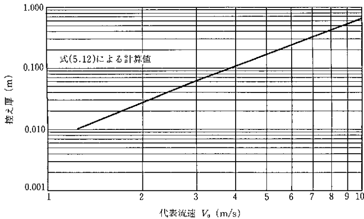
図参-25 連節型ブロックを用いたすりつけ護岸の控え厚の計算例
