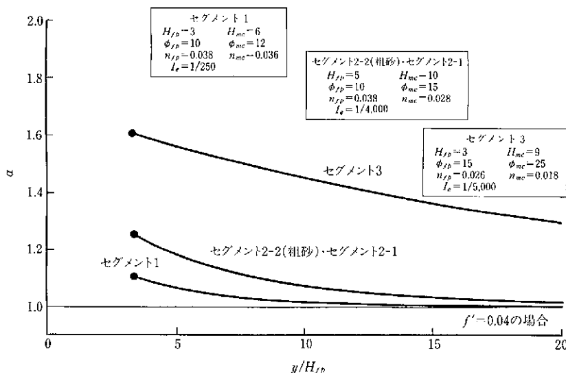
図4-8 高水護岸部の補正係数 \alpha と低水路法肩からの距離・高水敷水深比 ( y/H_{fp} ) との関係
