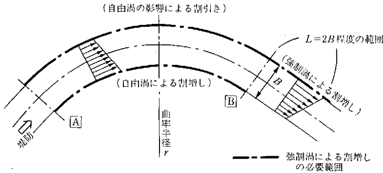
図4-10 堤防湾曲部の補正
