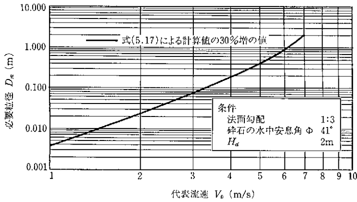
図参-31 代表流速 V_0 と必要な石の径 D_m の関係(3)
