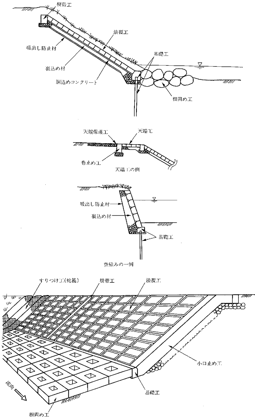
図 1-2 各部の名称
