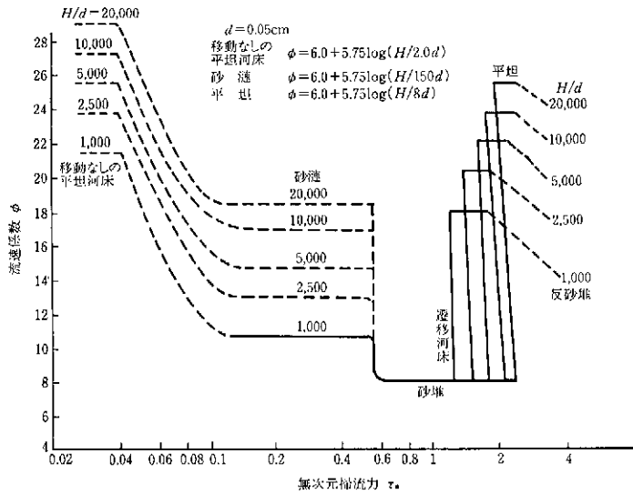
図参-7 \phi と \tau_* の関係 ( d=0.05\text{ cm} , H_d/d_R=1,000\sim 2,000 )
