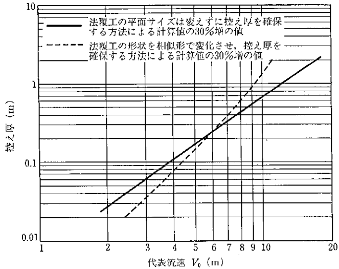
図参-24 練張り護岸を用いた天端保護工の控え厚 (平張りブロック)
