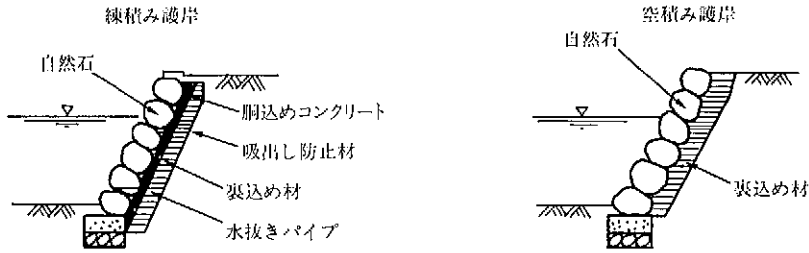
図5-25 土圧・水圧による滑動、転倒を対象とする積み護岸のモデル図
