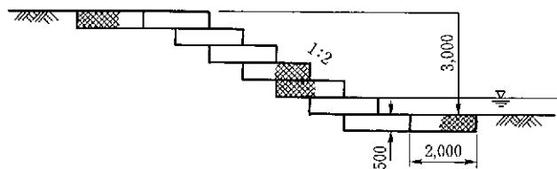
図参-33 布団籠工を階段状に設置した場合
