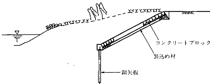
図 5-13 「滑動-群体」モデル工種のイメージ図
