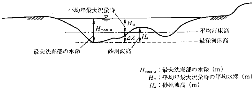
図 4-16 尖河川の最大洗掘部の水深 ( H_{max,s} ) の説明図
