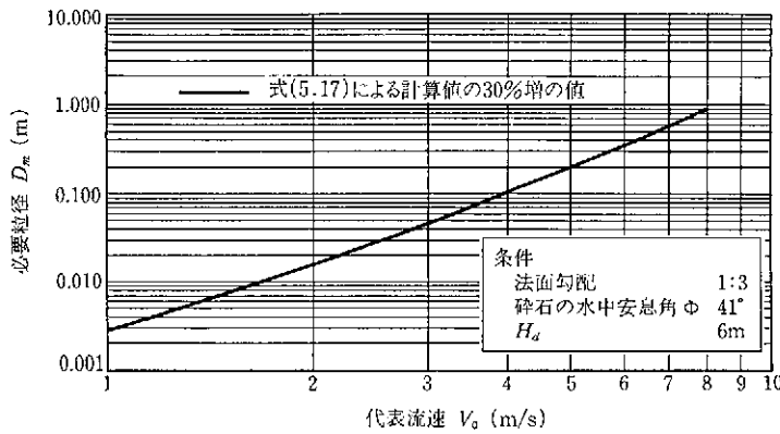
図参-32 代表流速 V_0 と必要な石の径 D_m の関係(4)
