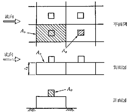
図参-39 護岸ブロックの水理特性試験法マニュアル（第2版）以前の「滑動-群体モデル」における投影面積の取り方
