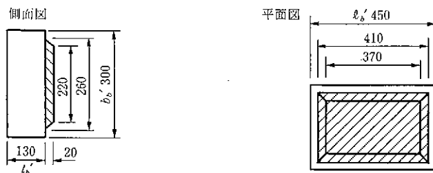
図参-17 平張りブロックの標準図
