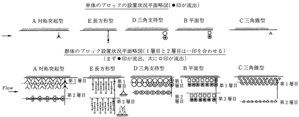
図 5-42 ブロック群の遮へい，かみあわせ効果実験模式図
