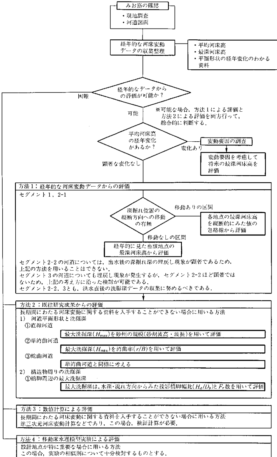
図4-12 最深河床高の評価方法の流れ
