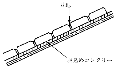
図5-10 破壊形態が滑動であり、群体として扱うことのできる法覆工のモデル図
