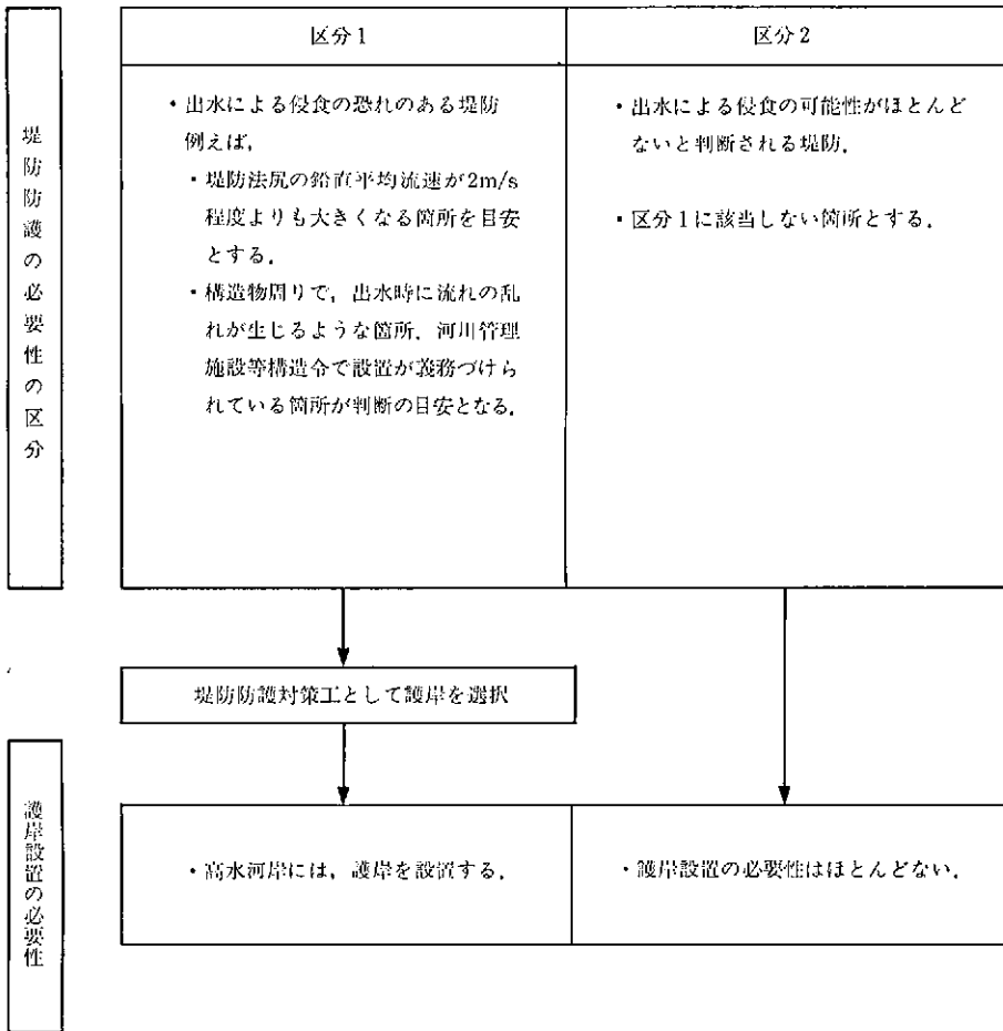
図2-8 堤防防護の必要性の区分と護岸設置の必要性
