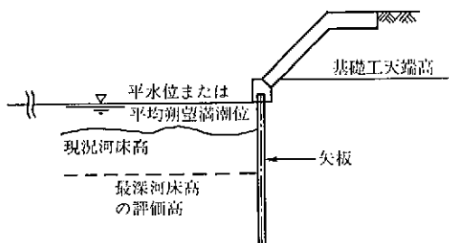
図 5-35 基礎の根入れが困難な場合の設置方法
