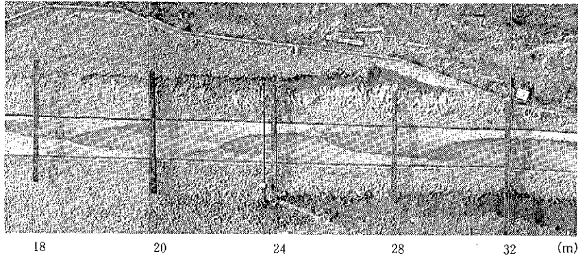
写真 4-1 被列砂州と交互砂州の共存 1)
