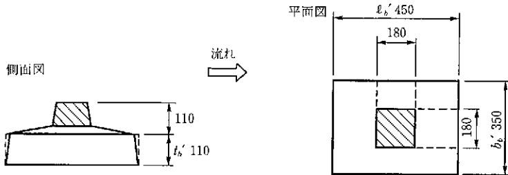
図参-21 連節型ブロックの標準図
