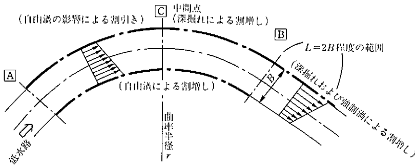
図4-9 移動床低水路の補正
