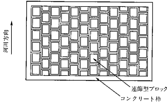
図参-22 群体として設置した場合の連節型ブロック
