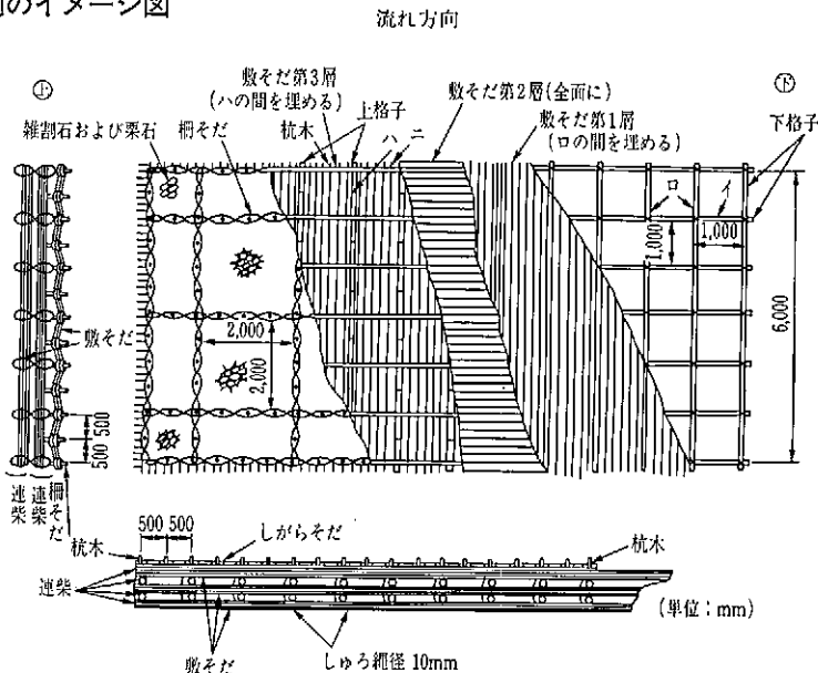
図 5-52 そだ沈床
