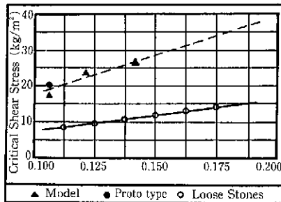
図5-23 籠詰め状態での限界掃流力
