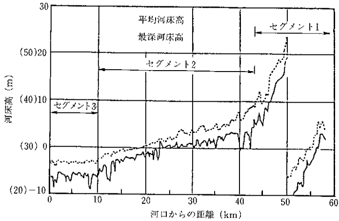
図2-2 木曾川平均河床高および最深河床高縦断面図 1)
