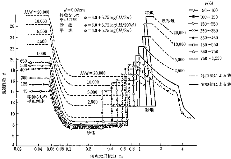
図参-8 \phi と \tau_* の関係 ( d_R=0.02\text{ cm} )
