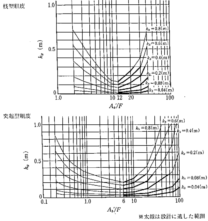
図参-11 h_g と A_0/F との関係
