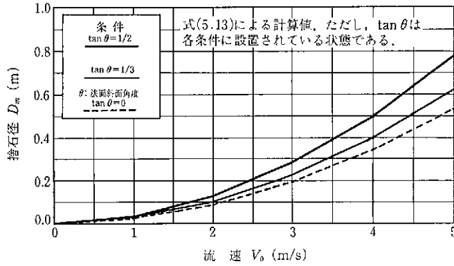
図参-27 代表流速 V_0 (m/s)で流失しない捨石径 D_m (m)の算定 (材料の水中安息角自然石, \Phi=38^\circ )
