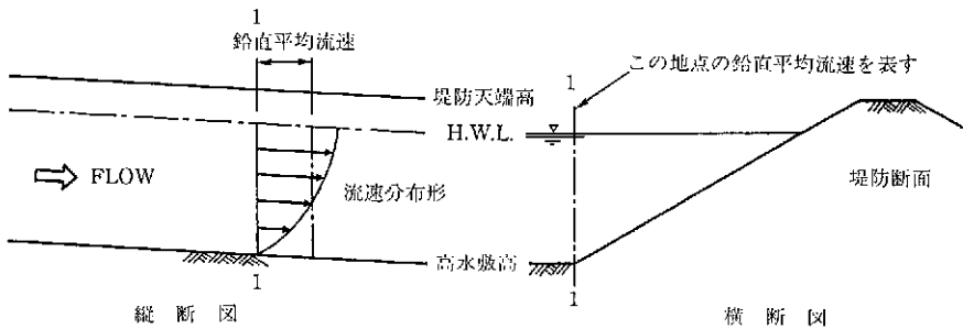
図2-6 堤防法尻位置の鉛直平均流速
