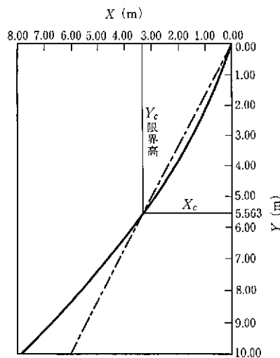
図参-37 練り積み護岸の中心線と示力線との関係
