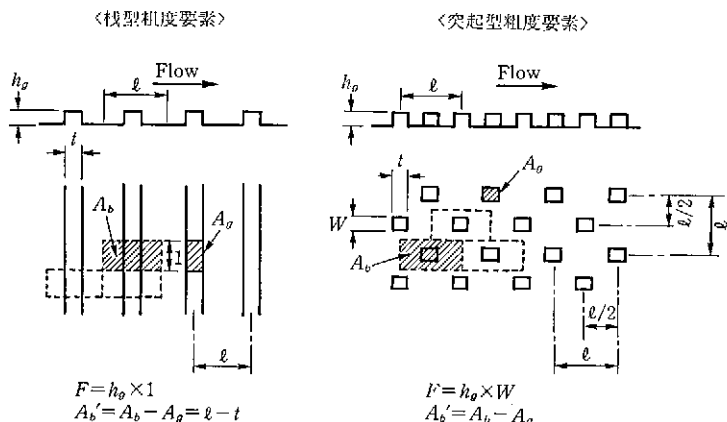
図参-10 粗度要素形状の定義
