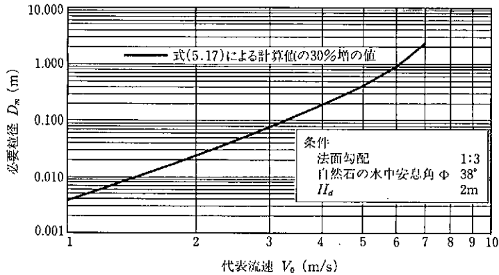
図参-29 代表流速 V_0 と必要な石の径 D_m の関係(1)
