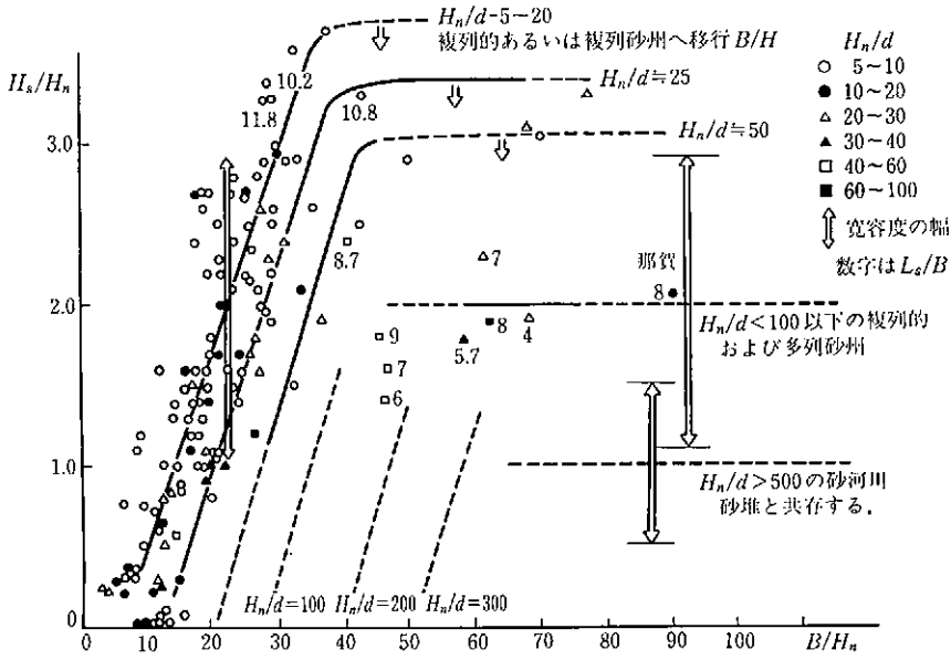
図 4-15 H_s/H_n と B/H_n の関係 (ただし \tau_* は 0.03~0.4 の範囲) 1)
