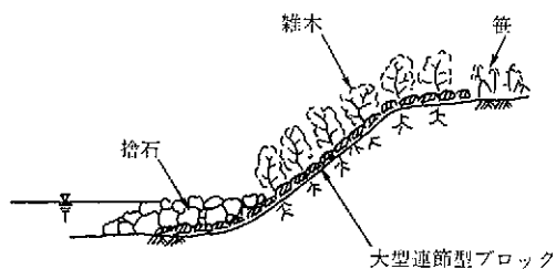
図5-17 めくれモデル工種のイメージ図
