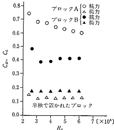
図5-7 単体ブロックの C_D 、 C_L
