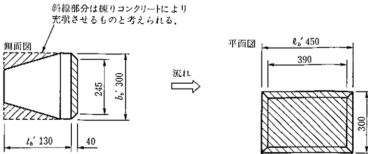
図参-19 間知ブロックの標準図
