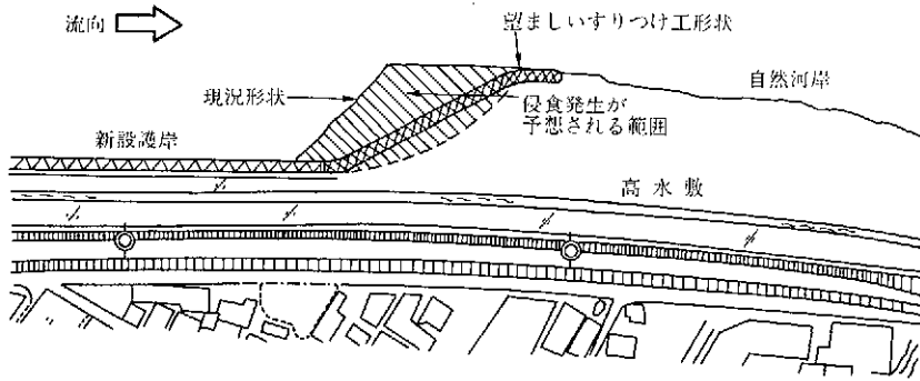
図2-9 すりつけ部の形状
