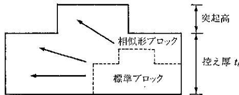
図5-6 スケール比 S で控え厚 t_b を確保する方法
