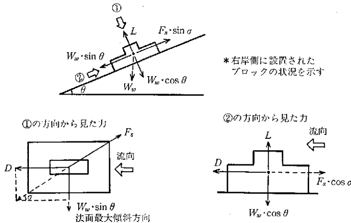
図5-3 力のつりあいモデル図
