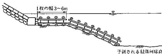
図5-37 重ね合わせない場合の敷設幅 (図は、そだ沈床の事例)
