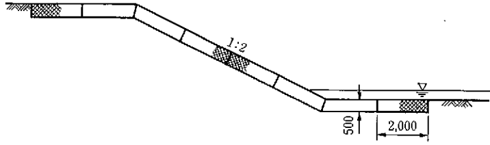
図参-34 布団籠工を斜面に設置した場合
