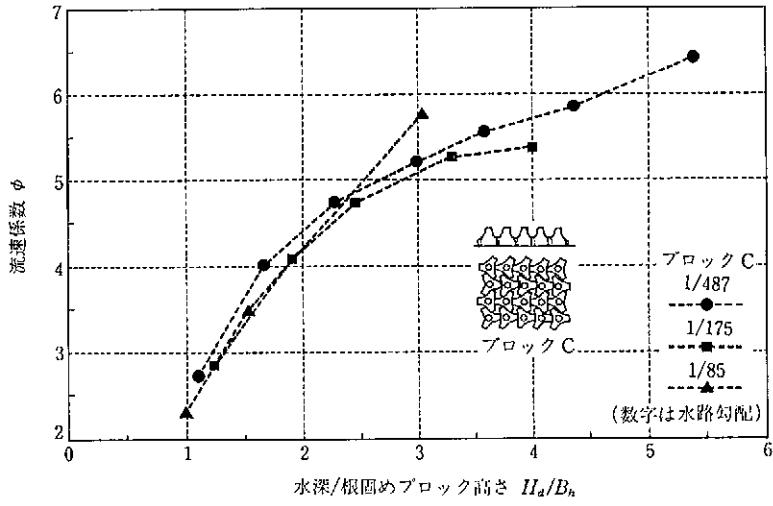
図参-14 流速係数 (ブロック C)
