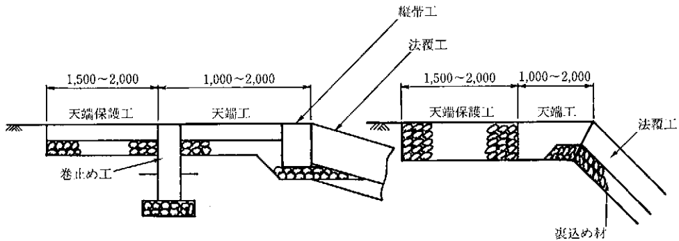
図5-29 天端工の幅 (設置例)
