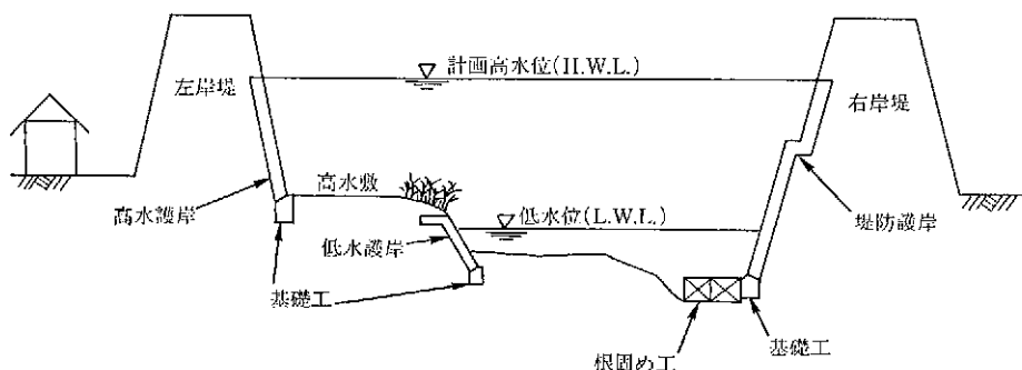
図 1-1 適用護岸種類説明図
