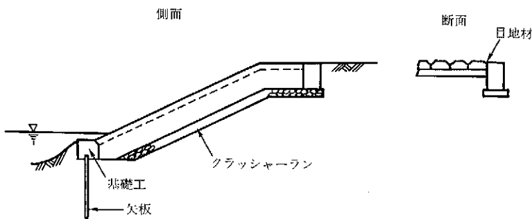
図5-30 小口止め工の例
