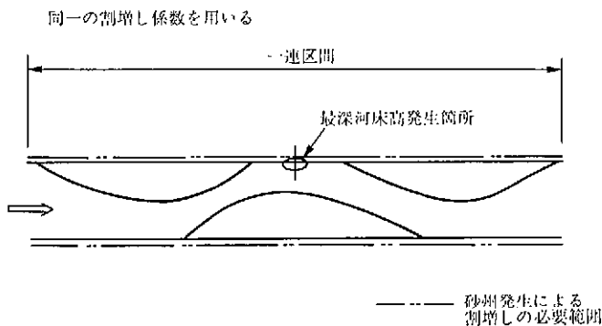
図 4-5 直線河道低水路の補正
