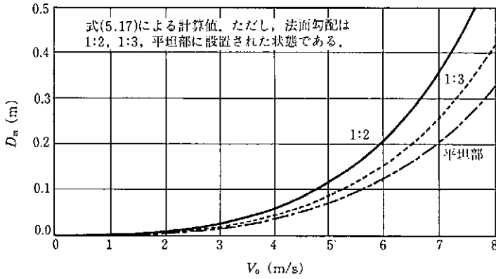
図参-36 D_m と V_0 の関係 (碎石の場合; \Phi=41^\circ ) の計算例
