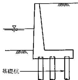
図5-27 土圧・水圧による滑動，転倒を対象とする擁壁護岸のモデル図
