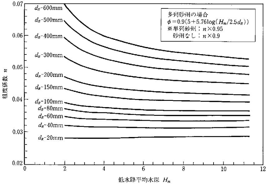
図参-2 セグメントの低水路粗度係数 ( I_b > 1/250 )
