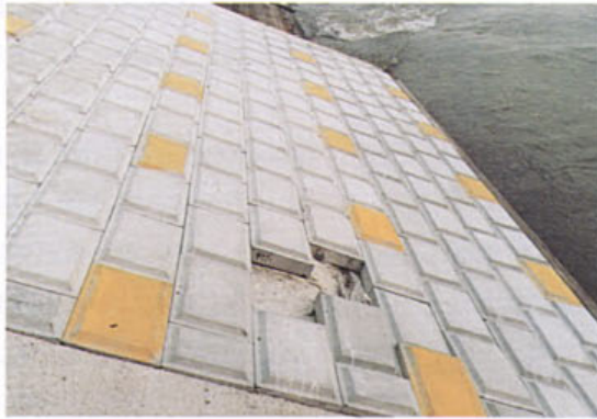
写真2-5 法覆工の被災事例
