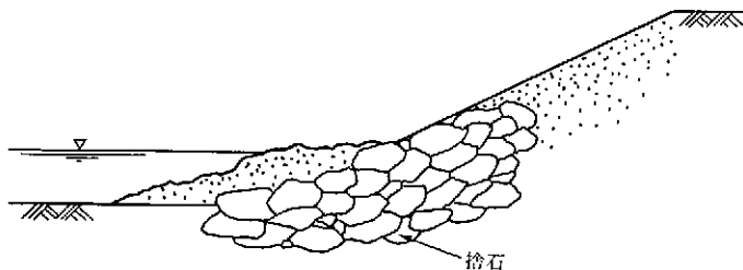
図 5-48 捨石根固め工
