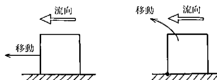
図5-41 安定条件図
