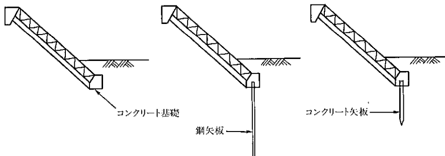
図 5-36 基礎工の工種例
