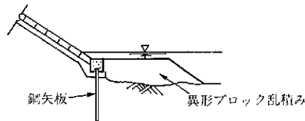
図 5-46 異形ブロック乱積み根固め工
