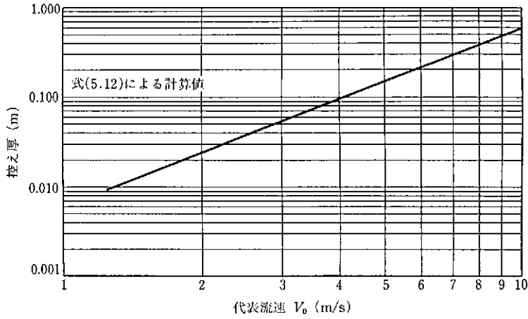
図参-26 連節型ブロックを用いた天端保護工の控え厚の計算例
