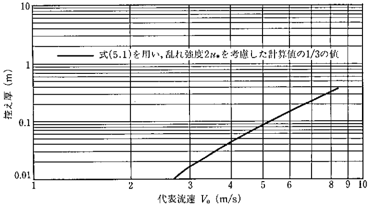
図参-15 平張りブロックの計算例 ( H_d=2 mの場合)
