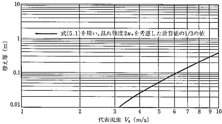
図参-16 平張りブロックの計算例 ( H_d=6 mの場合)
