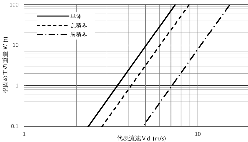
図参-38 平面型根固めブロックの流速と重量の関係の計算例
