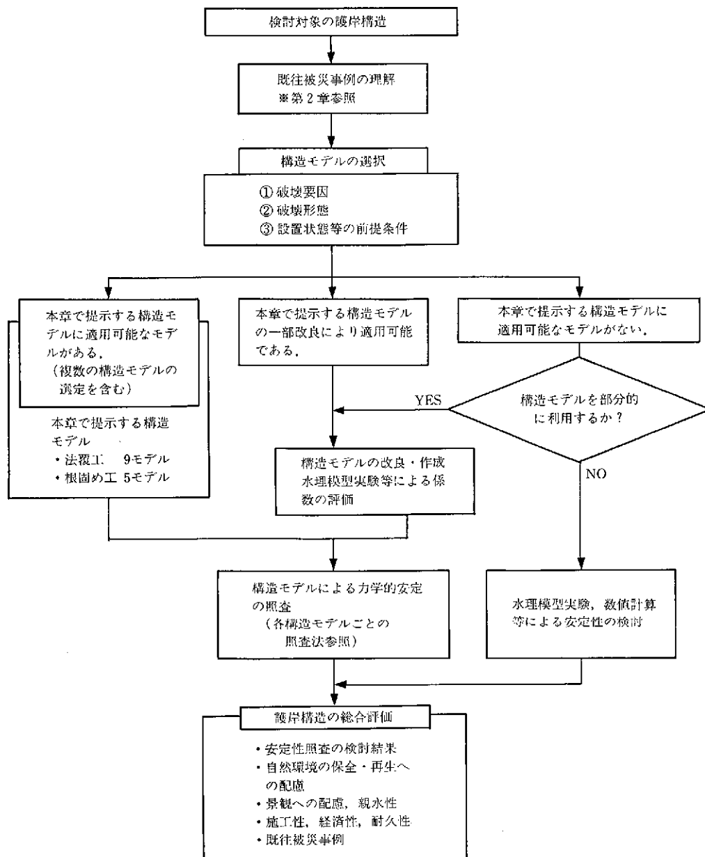
図 5-1 護岸の力学的安定性の照査手順
