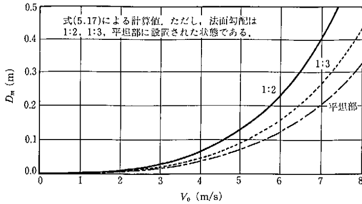
図参-35 D_m と V_0 の関係 (自然石の場合; \Phi=38^\circ ) の計算例
