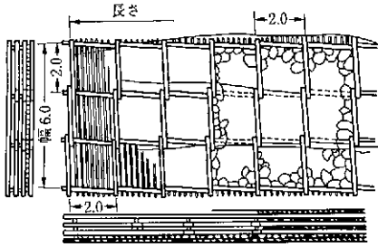
図5-53 木工沈床（4層建）
