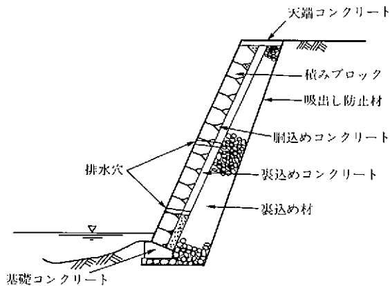
図5-31 裏込め材の設置例
