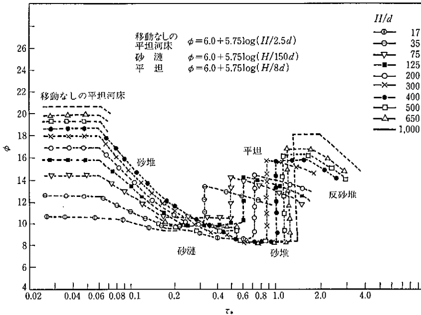
図参-1 \phi と \tau_* の関係 ( d_R が0.4 cm以上)
