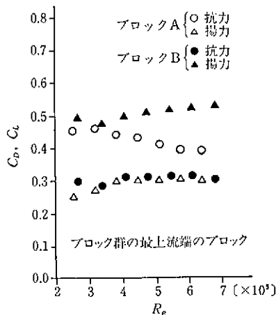
図 5-16 ブロック群最上流端ブロックの C_D , C_L
