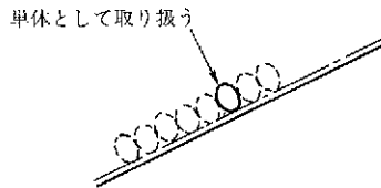
図 5-20 破壊形態が掃流であり一体性が強い法覆工のモデル図
