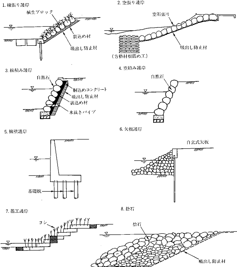
図 2-10 護岸工種例
