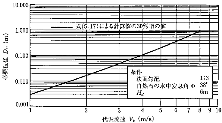
図参-30 代表流速 V_0 と必要な石の径 D_m の関係(2)
