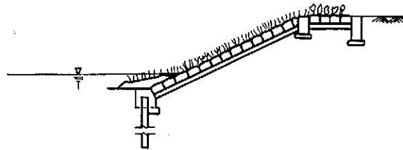
図5-9 「滑動単体」モデル工種のイメージ図
