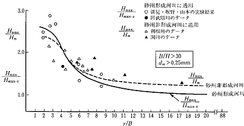
図 4-17 湾曲部における H_{max}/H_{max,s}(H_m) と r/B との関係 1)
