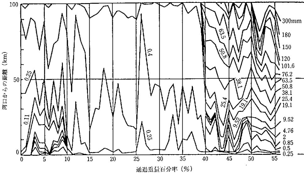
図 2-3 木曾川河床材料粒度分布変化図 1)
