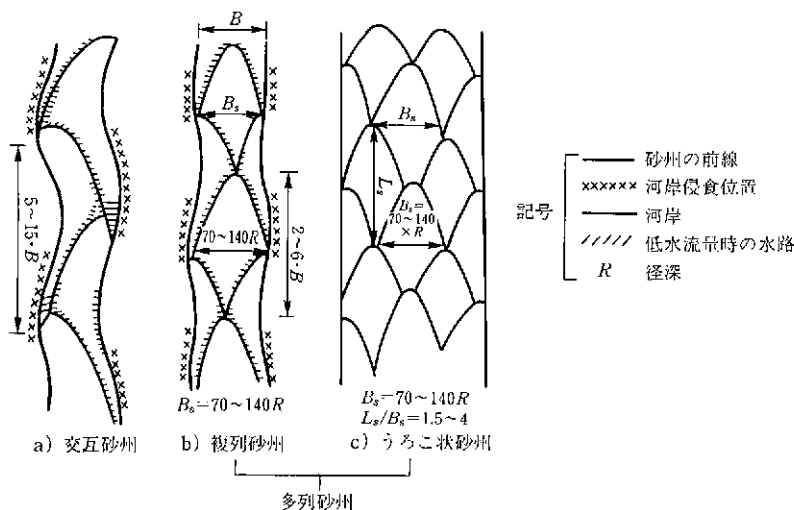
図 4-11 典型的な砂州のスケール 1)
