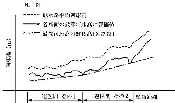
図4-13 洗掘部が縦断的に移動する河道の最深河床高の評価
