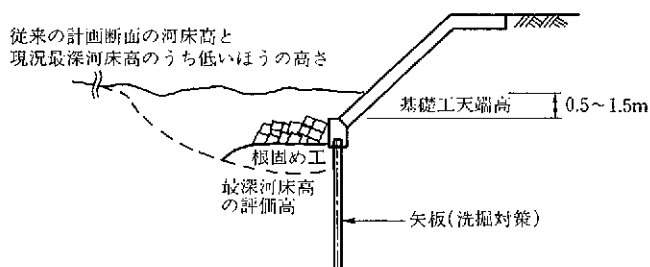
図5-34 基礎に矢板を併用する方法
