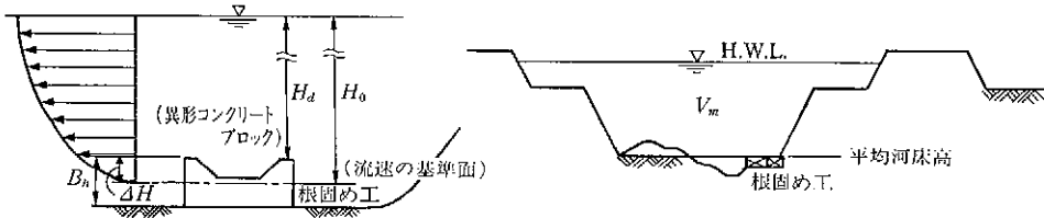
図参-12 根固め工上の水深のとり方
