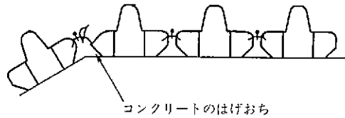
図5-43 ブロックの連結方法
