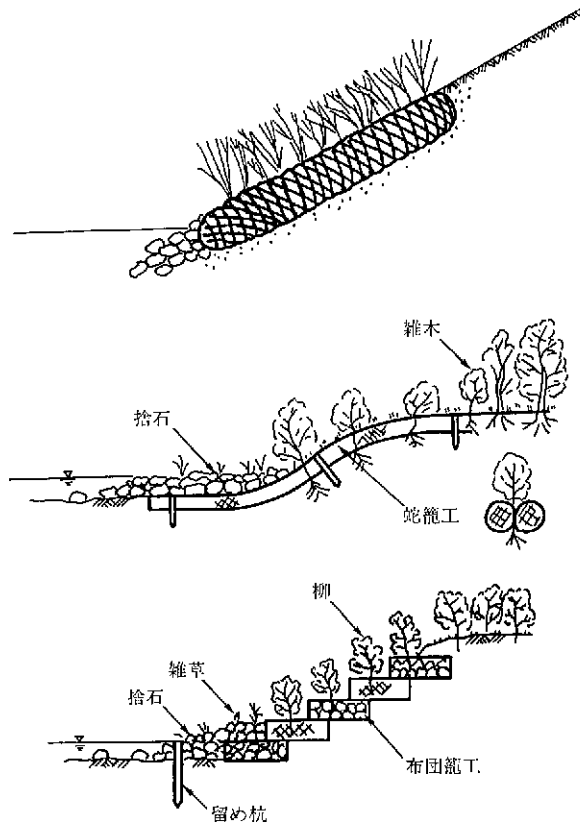
図5-24 「掃流-籠詰め」モデル工種のイメージ図
