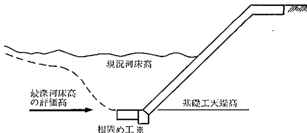
図 5-32 最深河床高の評価高を基礎工天端高とする方法
