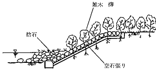
図 5-21 「掃流-一体性が強い」モデル工種のイメージ図
