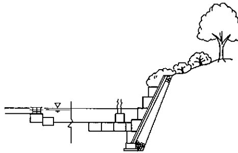
図5-26 「積み」モデルの工種イメージ図
