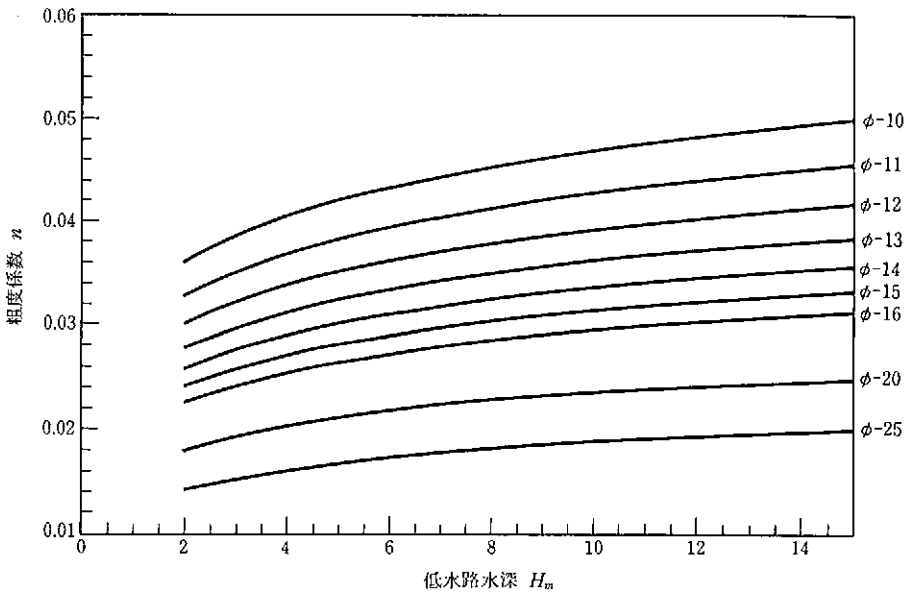
図参-4 n と H_m , \phi の関係
