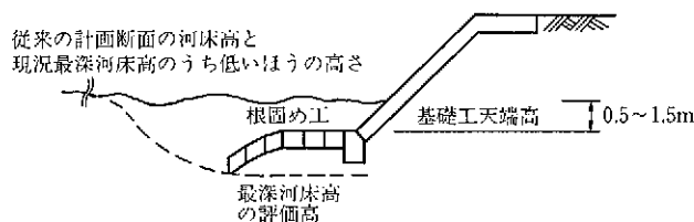
図5-33 根固め工で対処する方法
