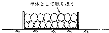
図 5-51 掃流を破壊形態とし中詰め状態の根固め工のモデル図
