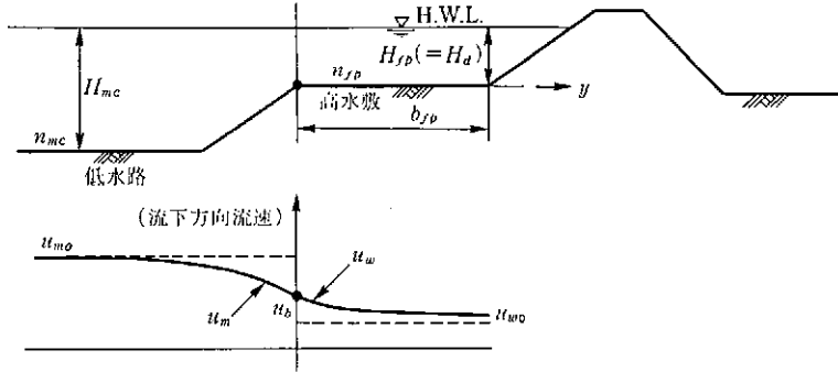
図 4-7 鉛直平均流速の横断分布
