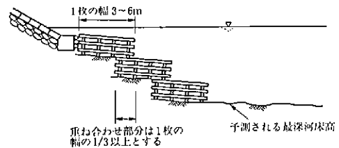
図5-38 重ね合わせる場合の敷設幅 (図は、木工沈床の事例)
