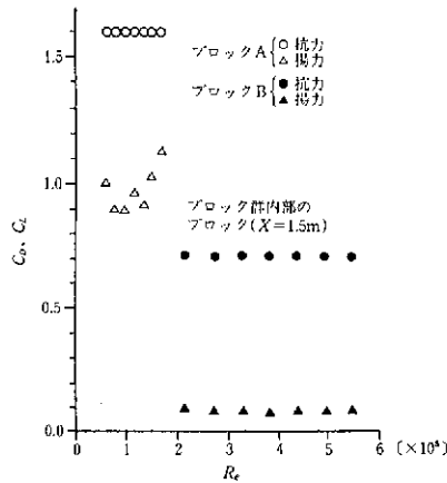
図参-40 上記条件におけるブロック群内部の抗力係数と揚力係数
