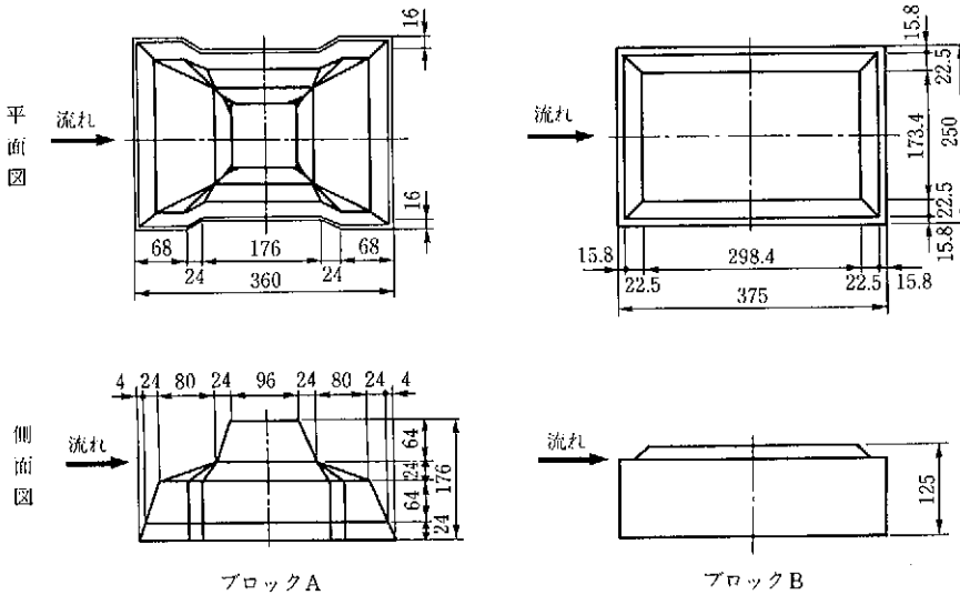
図5-8 ブロック標準図
