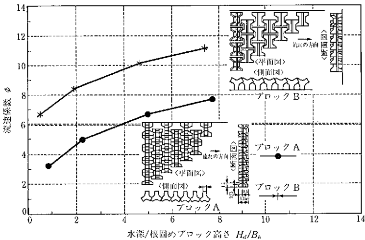
図参-13 流速係数（ブロックA, B）
