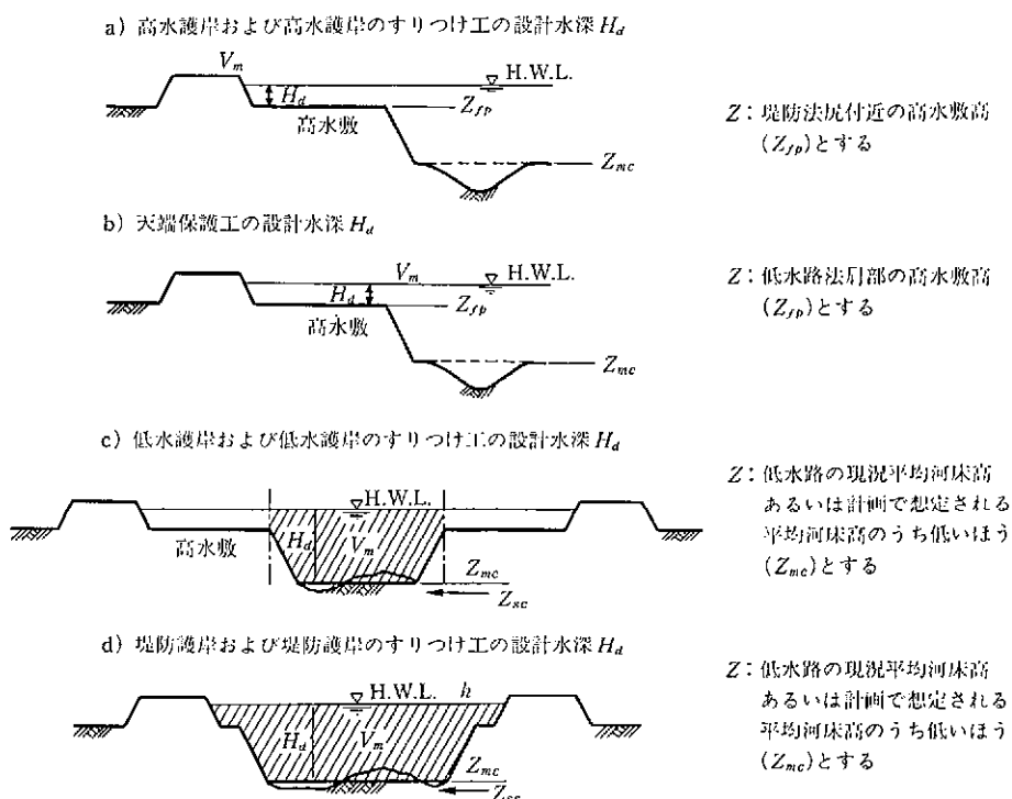
図 4-3 横断形状別に見た平均流速 V_m と設計水深 H_d の説明図
