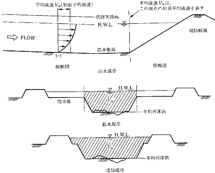
図4-2 平均流速 V_m の説明
