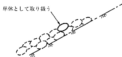
図 5-47 掃流を破壊形態とする乱積み状態の根固め工のモデル図
