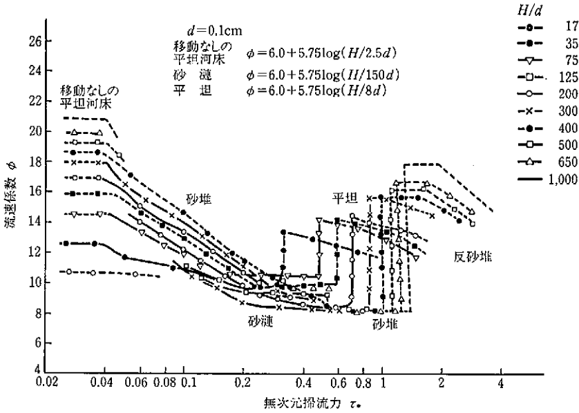
図参-5 \phi と \tau_* の関係 ( d=0.1 cm, H_d/d_R=15\sim1,000 )
