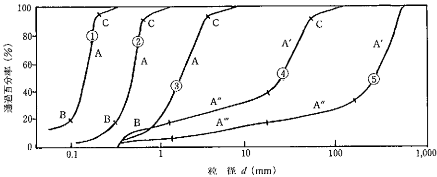
図2-1 種々の粒度分布における縦断区分点 1)
