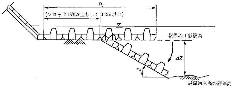
図5-39 滑動・転動を安定検討条件の対象とする根固め工の敷設幅
