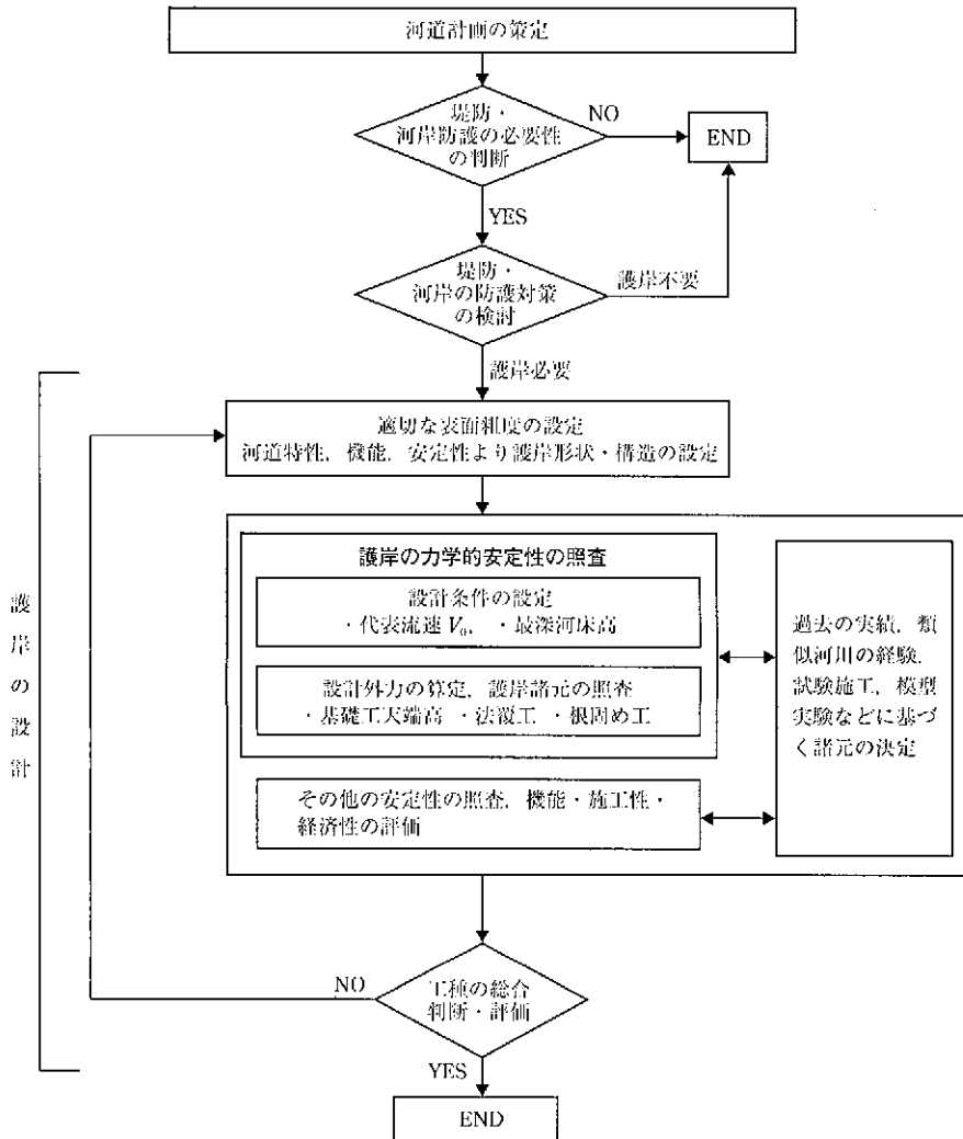
図 3-1 護岸の設計手順
