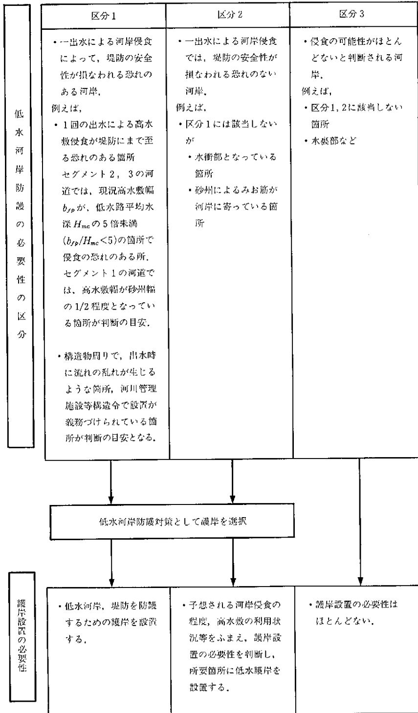
図2-7 低水河岸防護の必要性の区分と護岸設置の必要性
