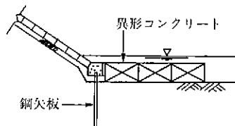
図5-44 異形ブロック層積み根固め工
