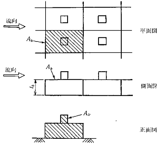
図5-4 投影面積の説明
