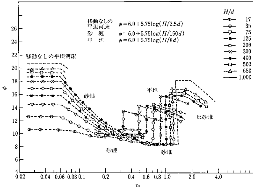
図参-3 \phi と \tau_* の関係 ( d_R が 0.4 cm 以上)
