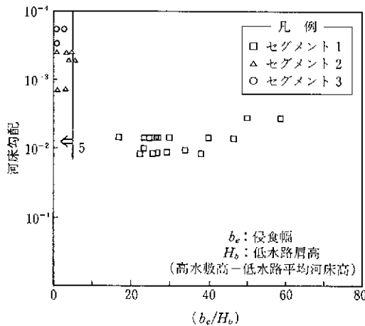
図2-4 侵食幅と河床勾配との関係 3)
