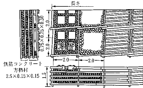
図5-54 改良木工沈床
