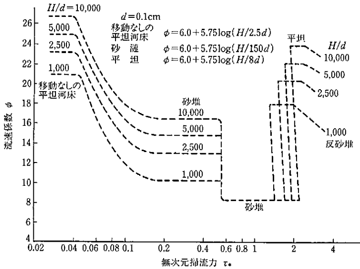
図参-6 \phi と \tau_* の関係 ( d=0.1 cm, H_d/d_R=1,000\sim10,000 )
