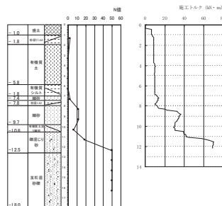
施工記録例
