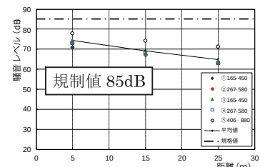
騒音レベル
