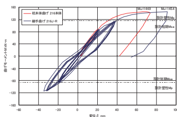
CCジョイント継手曲げ試験結果(HCCJ)
