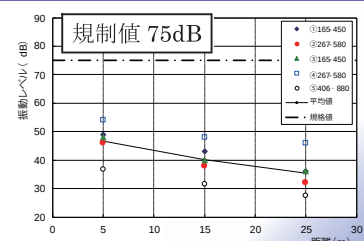
振動レベル
