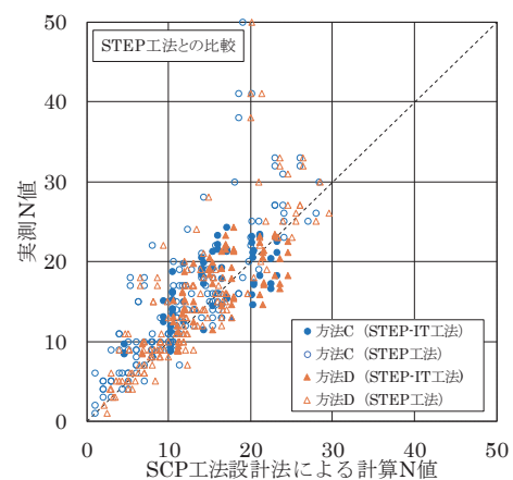
杭間の計算N値と実測N値の比較
