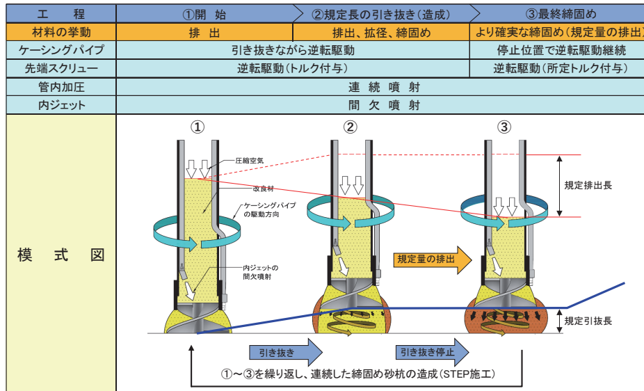
造成メカニズム
