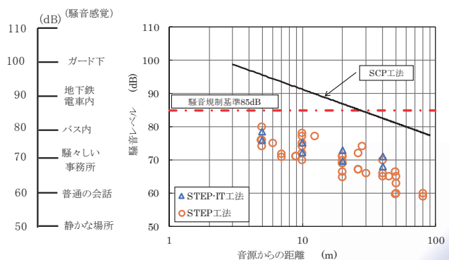
騒音レベルの確認結果
