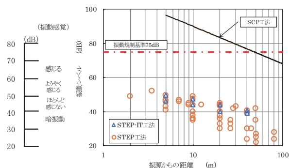
振動レベルの確認結果
