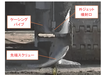
先端部構造
