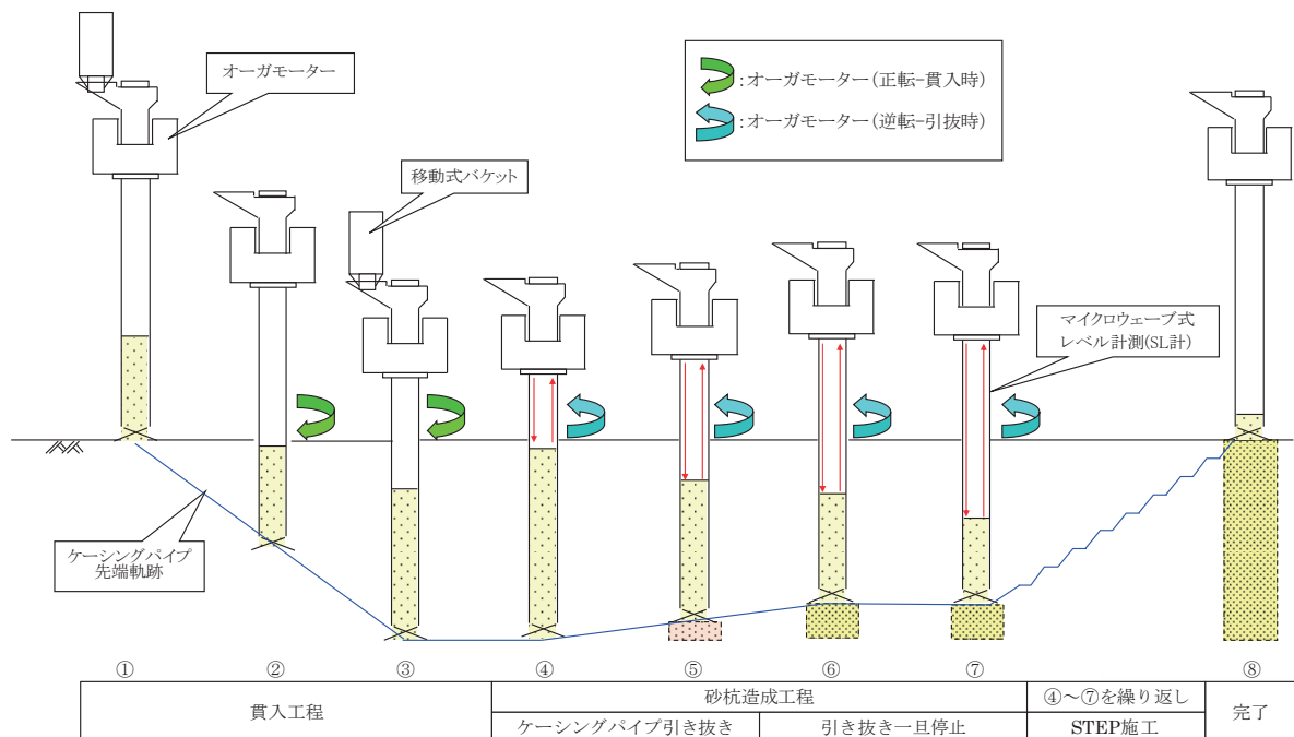
施工サイクル模式図
