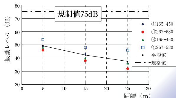
振動レベル
