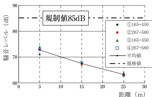
騒音レベル
