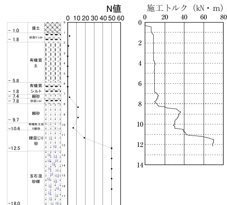
施工記録例
