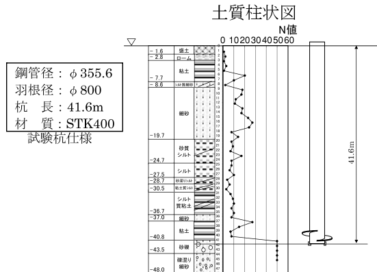
載荷試験概要(H-1 猿島)
