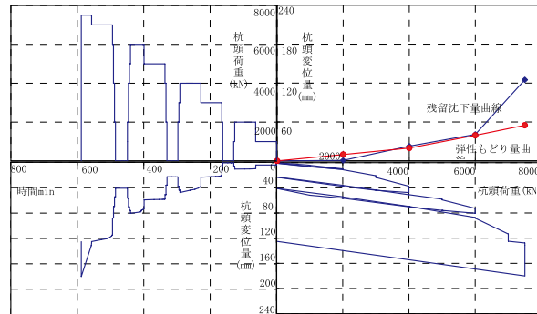
鉛直載荷試験結果
