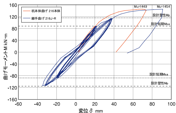
CCジョイント継手曲げ試験結果
