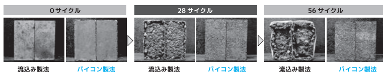
図－4 凍結融解試験
