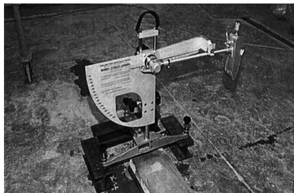
写真－3 滑り試験状況
