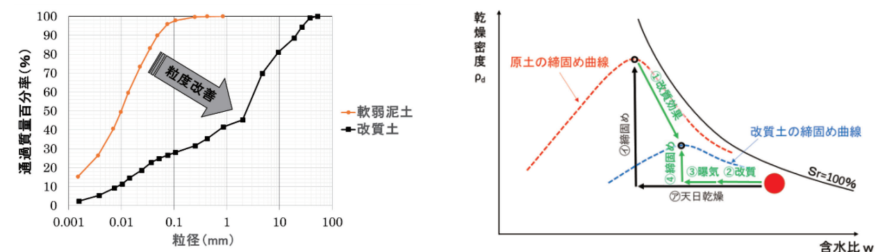
図－2 ほぐし造粒土の粒度改善特性
