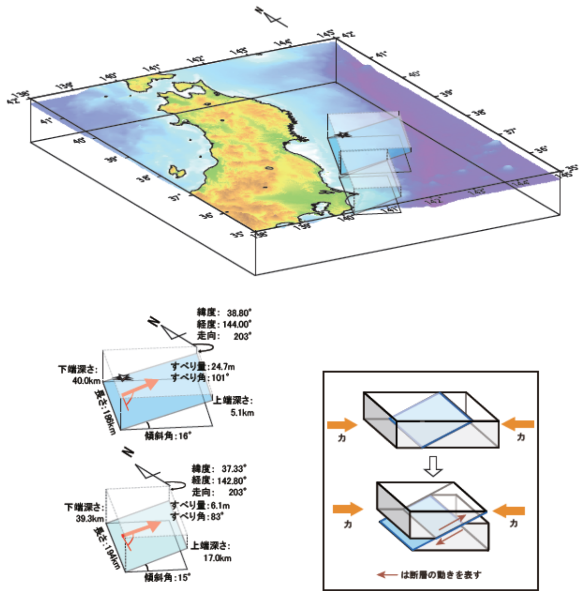
断層モデルのパラメータ
