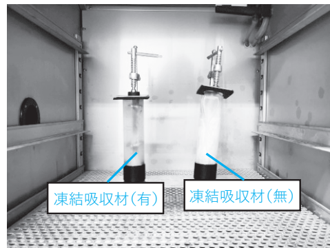
写真-4 凍結膨張吸収性能確認試験
