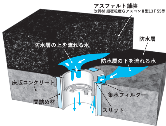
図－1 排水構造イメージ図
