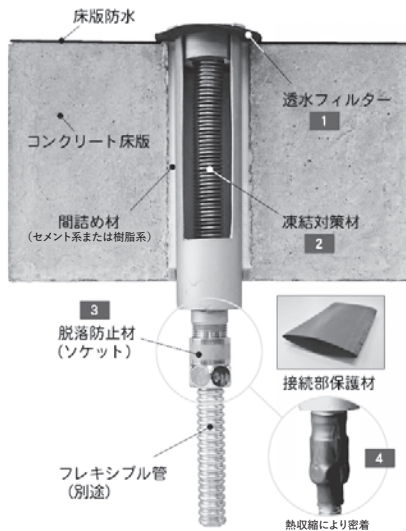
写真－5 高性能床版排水パイプ 概要
