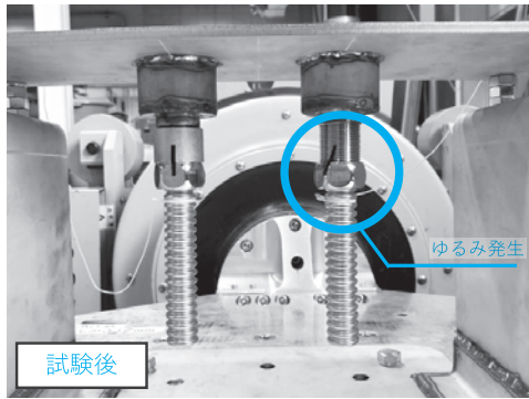
写真-2 脱落防止性能確認試験
